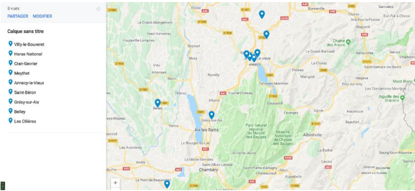
Carte 1 : Localisation des nids de frelon asiatique de 2018 pour le département de la Haute-Savoie
